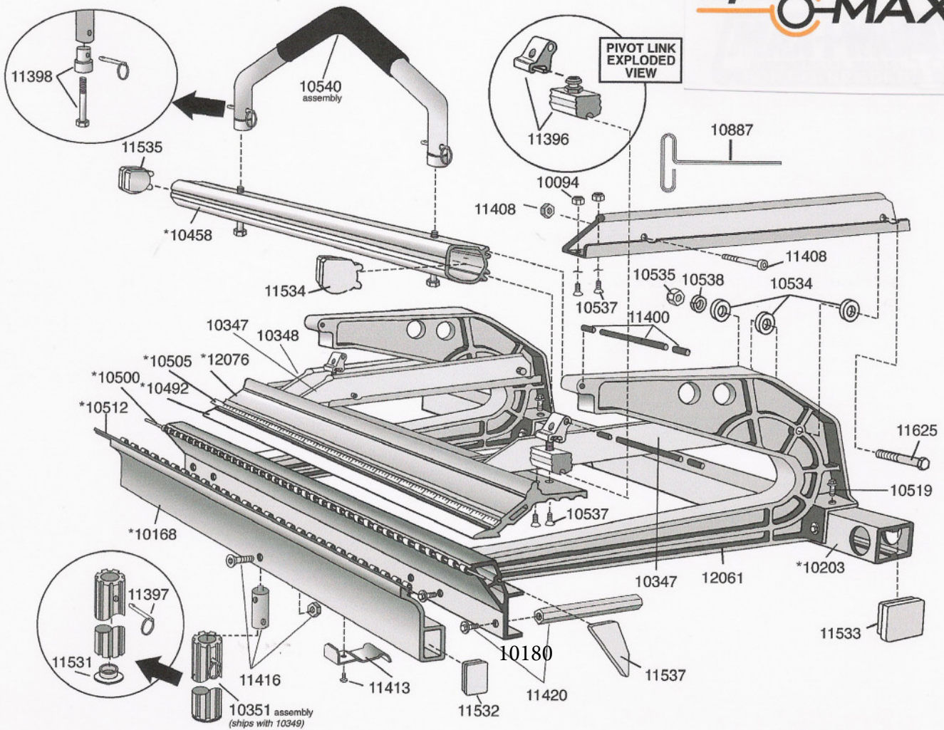
Na rysunku Numery części dla modelu Max 20 - 10
